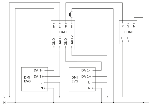
Schema elettrico Master-Master collegamento in rete
